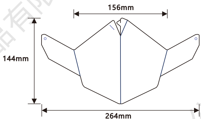
透明口罩展開尺寸
